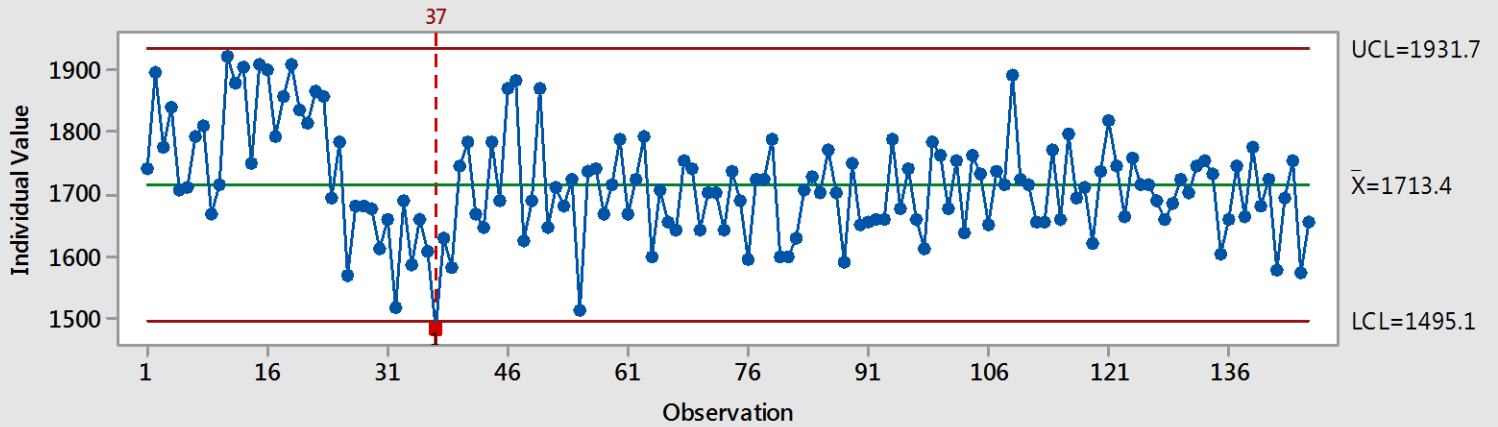
I-MR Chart of Gold Creek IM
